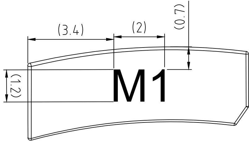
镭雕尺寸图（在凹面单面做此镭雕）
